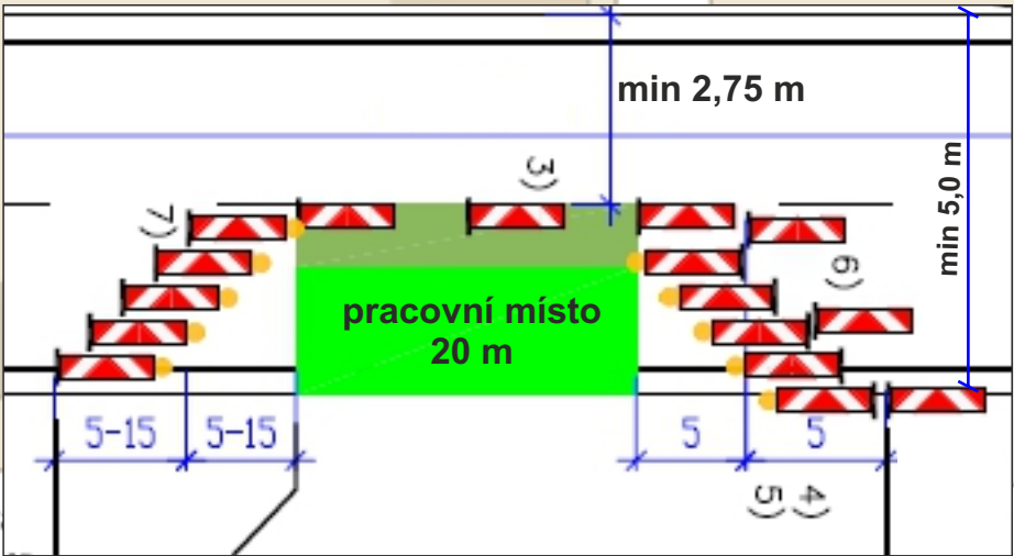
označení pracovního místa v jízdním pruhu
