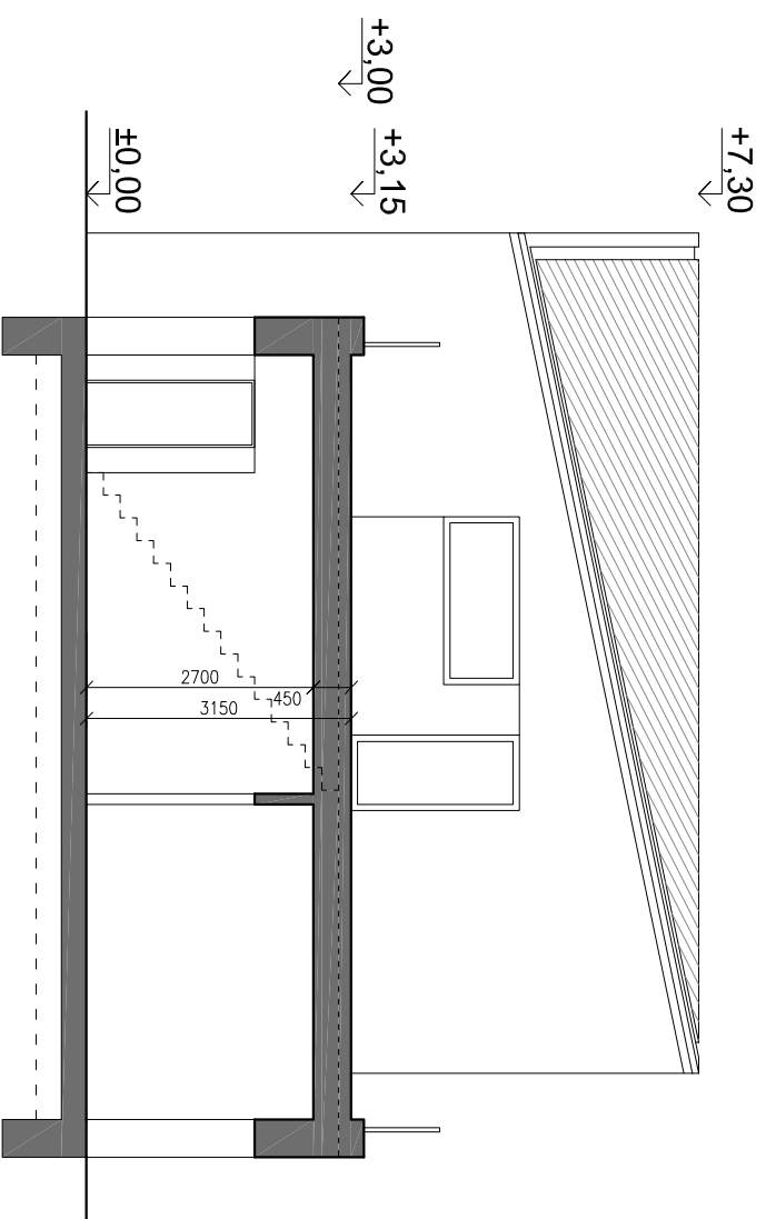
ŘEZ PODÉLNÝ
