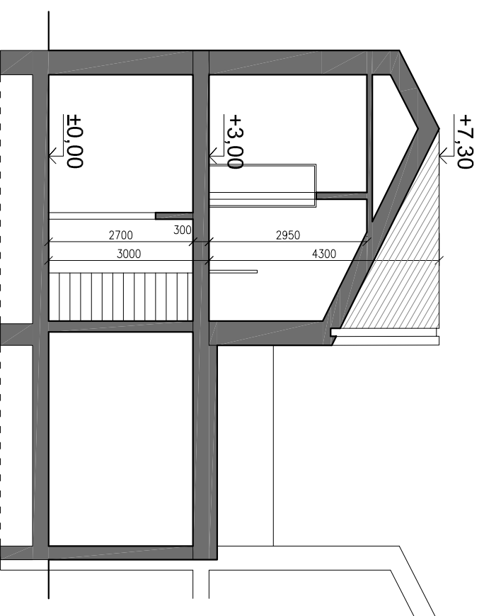
ŘEZ PŘÍČNÝ
