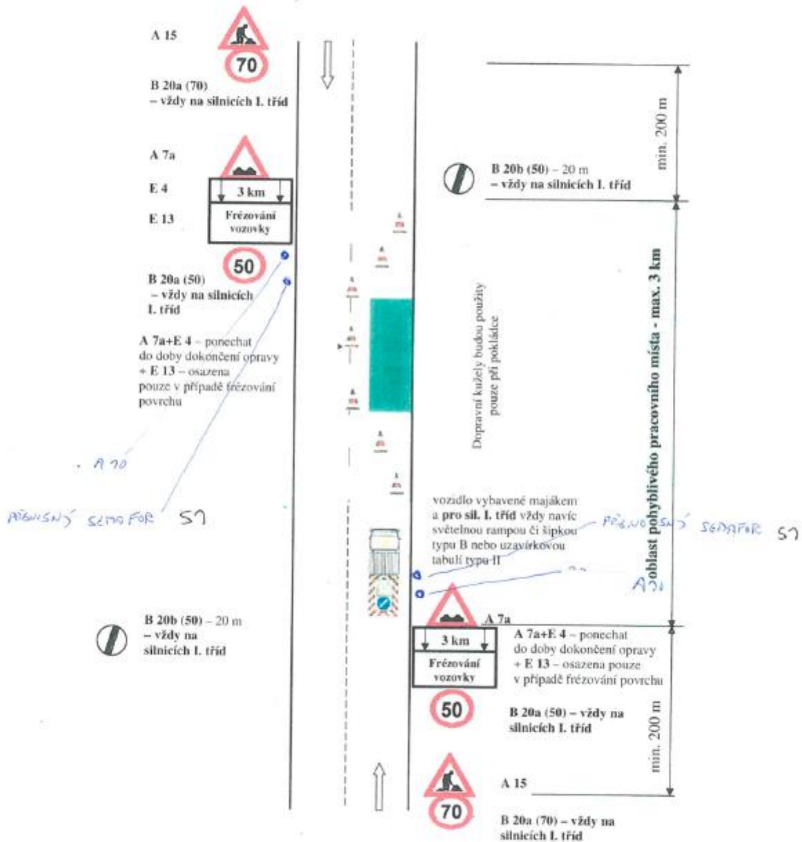
Schéma č. 2.2.: Výspravy vozovek obalovanou živičnou směsí s případným frézováním poruchy – mimo obec
