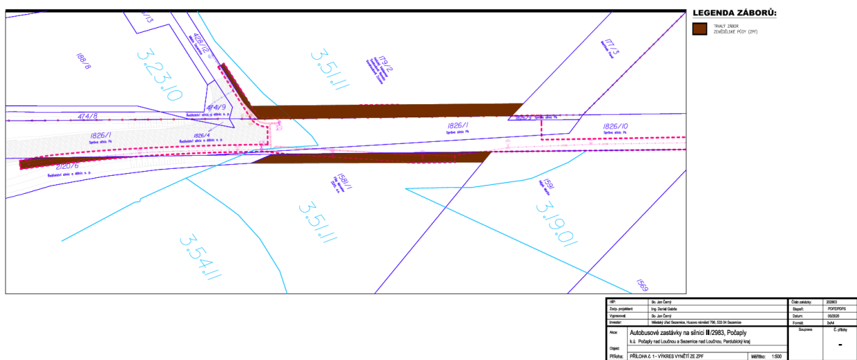
PŘÍLOHA č. 1 - VÝKRES VYNĚTÍ ZE ZPF 1:500
