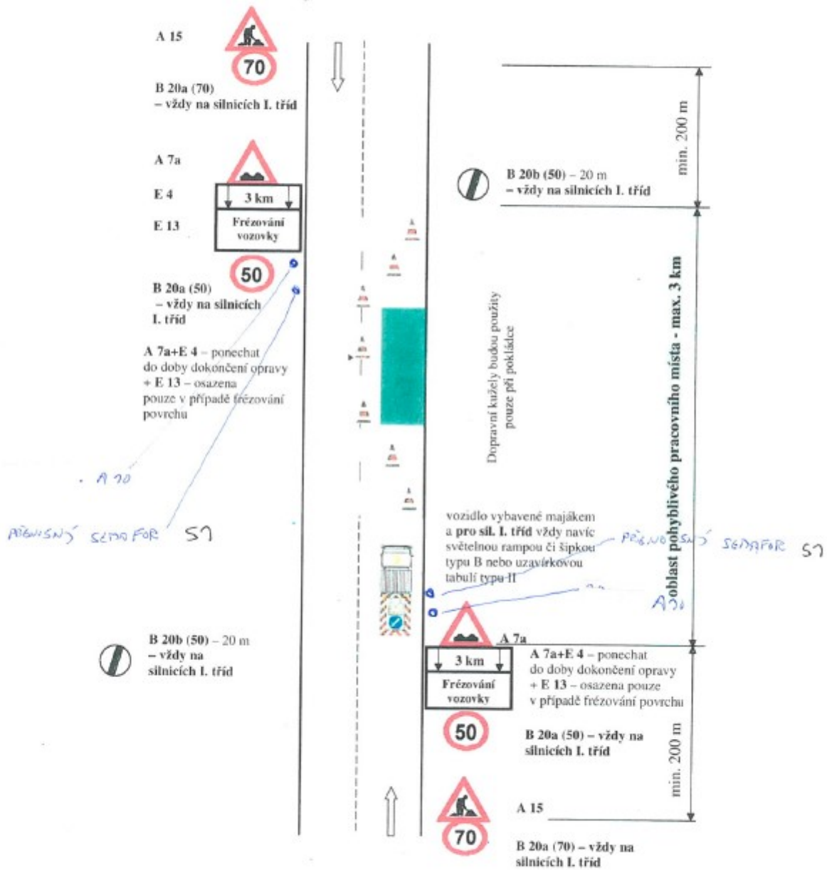
Schéma č. 2.2.: Výspravy vozovek obalovanou živícnou směsí s případným frézováním poruchy – mimo obec
