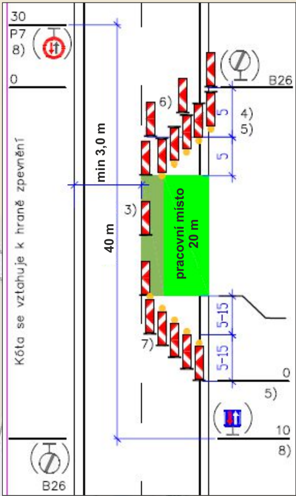
pohyb stavební techniky na komunikaci pouze v pracovní době, označení pracovního místa podle schéma OD 231
