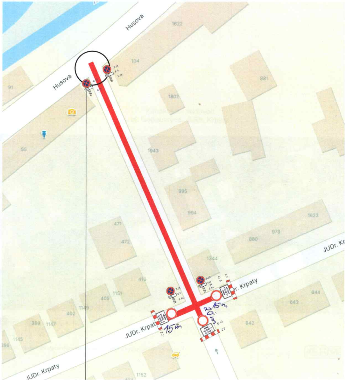
schéma B/5.2
