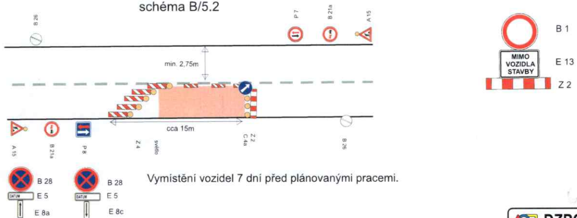
schéma B/5.2
