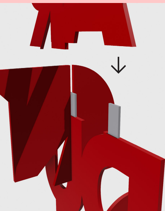
propojovací čepy ocel 8mm
