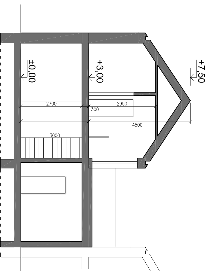
ŘEZ PŘÍČNÝ
