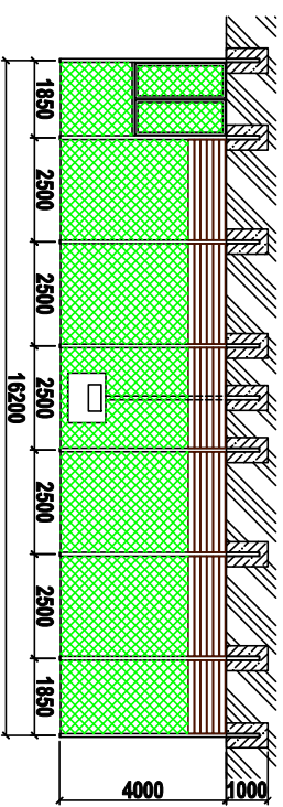
Pohled P3
